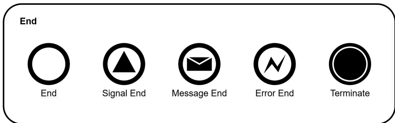
Eventos finales
