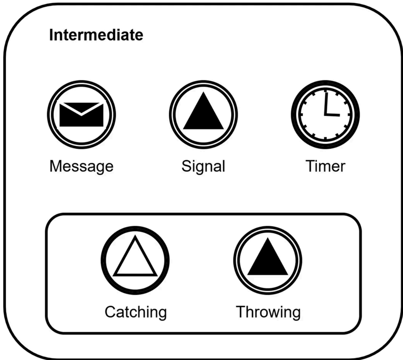
Eventos intermedios
